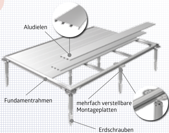
Abb. Erdschrauben-Fundament
